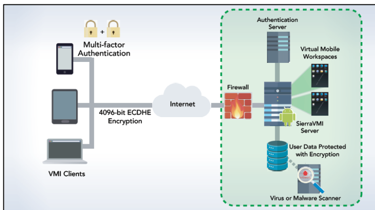
Abbildung 4: VMI-Technologie für Smartphones
