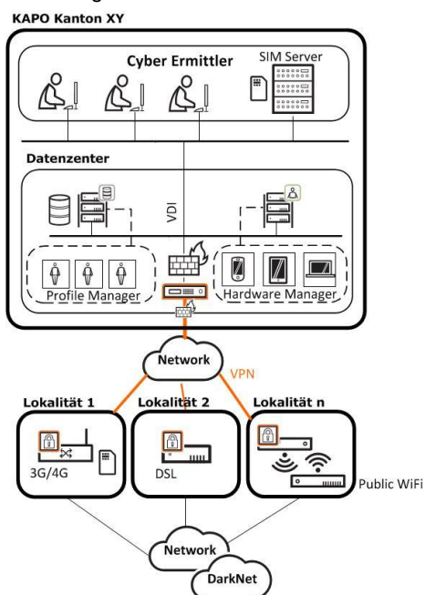
Abbildung 1: Schematische MINA-Architektur
